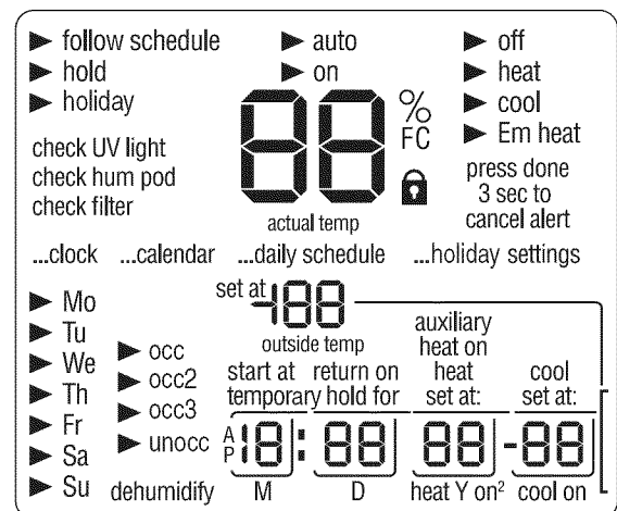
Fig. 1 — Thermostat Display
