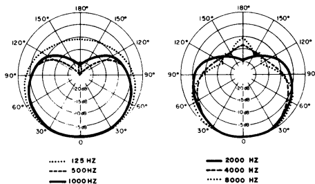
COURBES DE DIRECTIVITÉ TYPIQUES FIGURE 3
