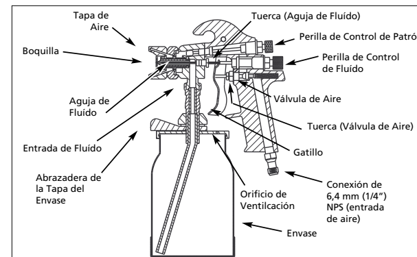
Figura 15 - Pistola Pulverizadora de Sifón
