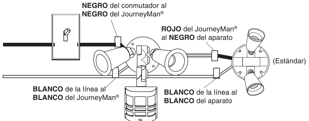
Conexión a la luz de movimiento y al aparato estándar
